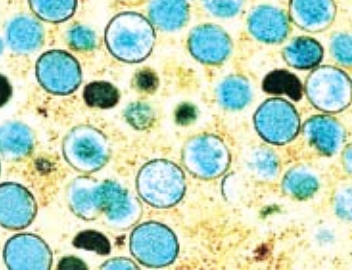
猴痘病毒
